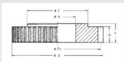
TYPE 45 - Zahnradbeschichtungen / Plating of gears
