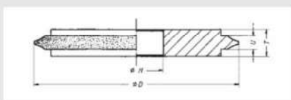
TYPE 44 - Zahnflankenschleifscheiben / Gear grinding wheels
